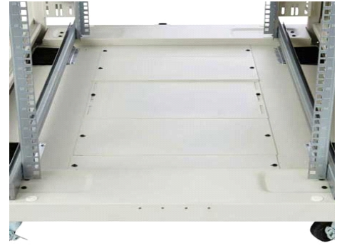
Accès des câbles par les panneaux amovibles de la base
