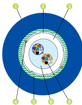
Construction en 16 Fibre
