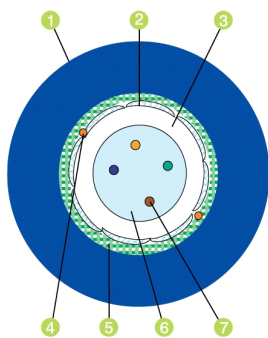
Construction en 4, 8 & 12 Fibres
