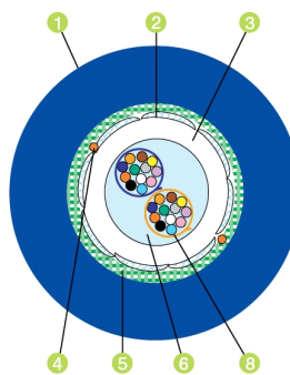
Construction en 24 Fibres
